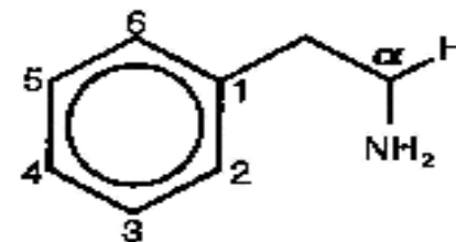
Fenetilaminai
